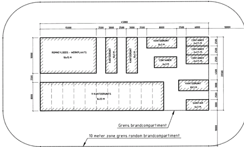
Voorbeeld 1. Terrein indeling m.b.v. éénlaagse bouw. Totaal brandcompartiment oppervlak: 910 m 2 enkel bestaande uit grondoppervlak: 910 m 2 Vrije afstandsgrens rondom: 10 m
