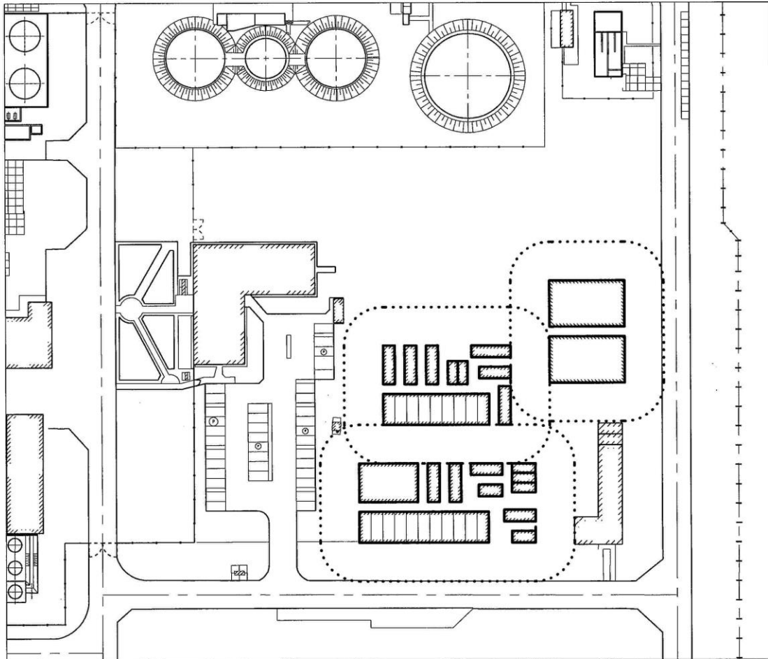
VOORBEELD INDELING CONSTRUCTIETERREIN MET GEBRUIKMAKING VAN BRANDCOMPARTIMENTEN
