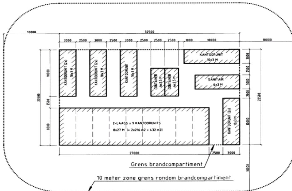
Voorbeeld 2. Terrein indeling m.b.v. één- en tweelaagse bouw. Totaal brandcompartiment oppervlak: 972 m 2 bestaande uit grondoppervlak: 666 m 2 + etages 306 m 2 Vrije afstandsgrens rondom: 10 m
